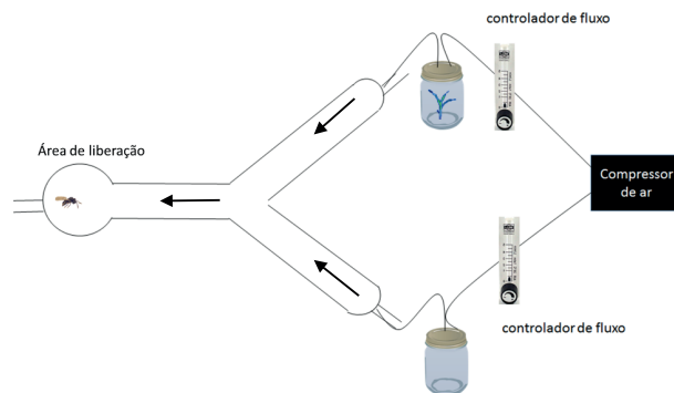
Figura 4. Desenho esquemático do olfatômetro em “Y” utilizado para testar a resposta do parasitoide de ovos Telenomus remus aos voláteis das plantas de milho. As setas indicam o sentido do fluxo de ar.
